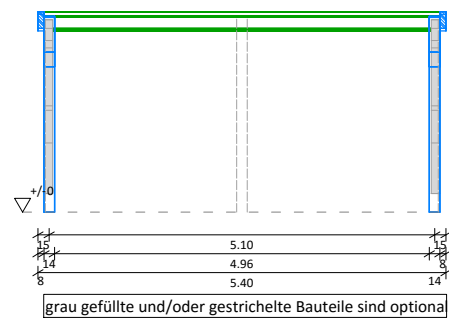
Schnitt: quer
