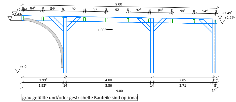
Schnitt: längs
