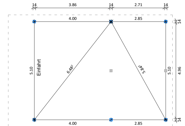
Horizontalschnitt: Pfostenmitte
