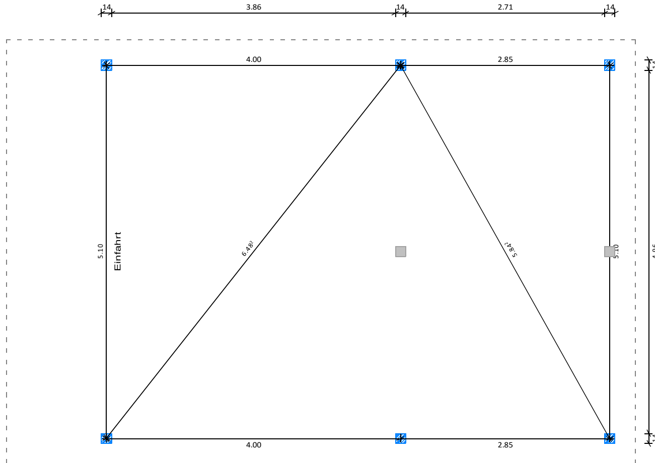
Horizontalschnitt: Pfostenmitte
