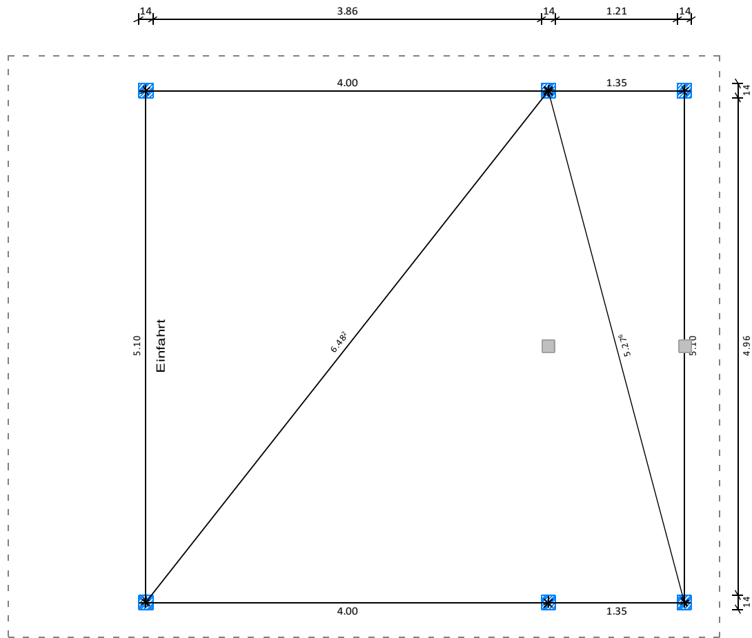
Horizontalschnitt: Pfostenmitte
