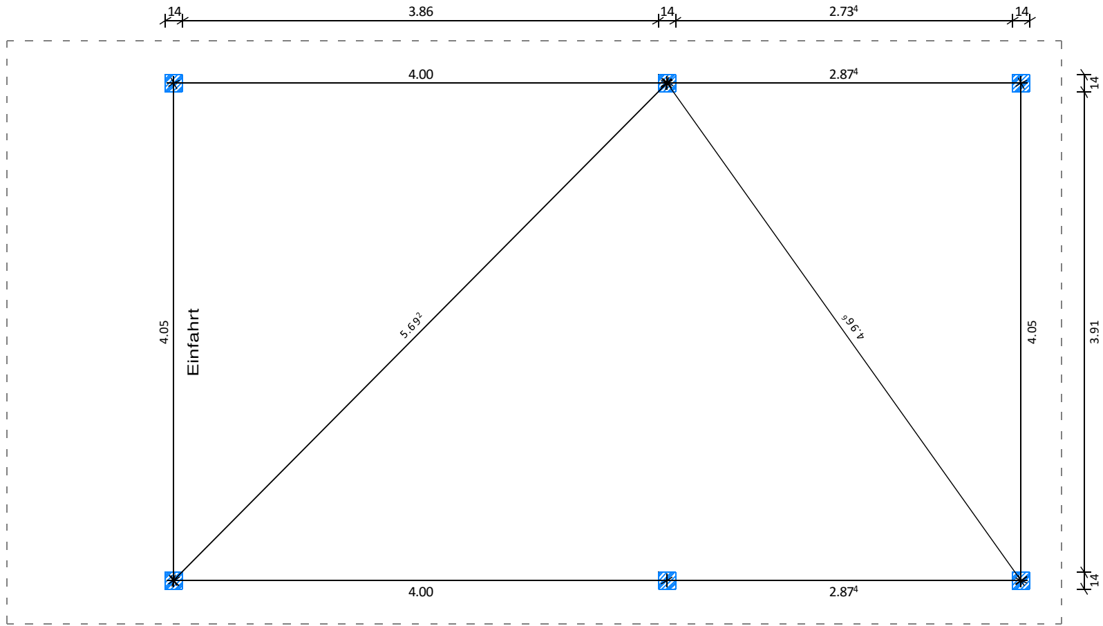
Horizontalschnitt: Pfostenmitte
