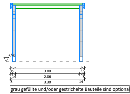
Schnitt: quer
