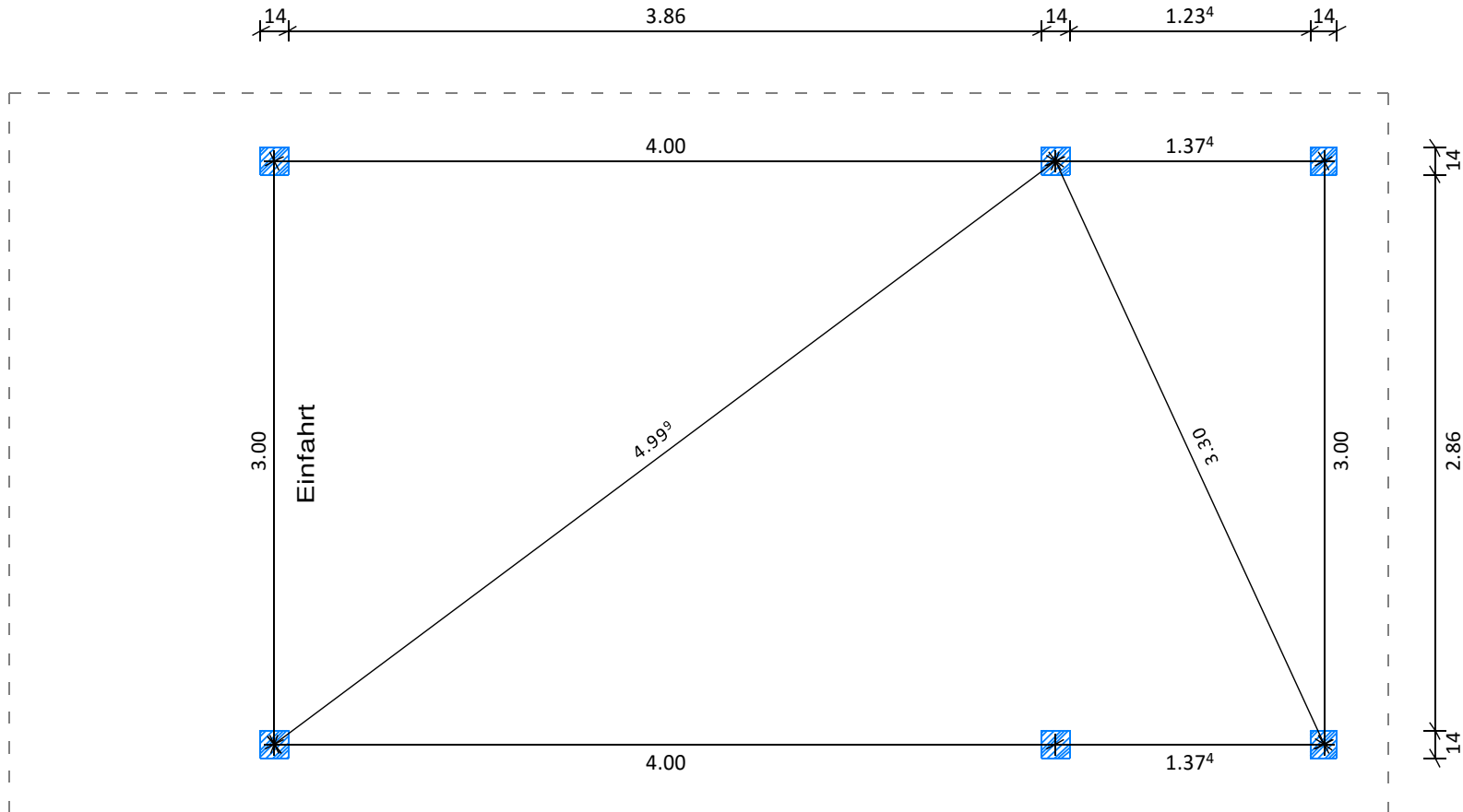
Horizontalschnitt: Pfostenmitte
