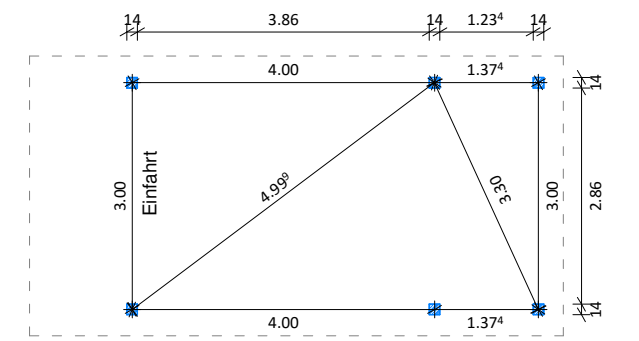
Horizontalschnitt: Pfostenmitte
