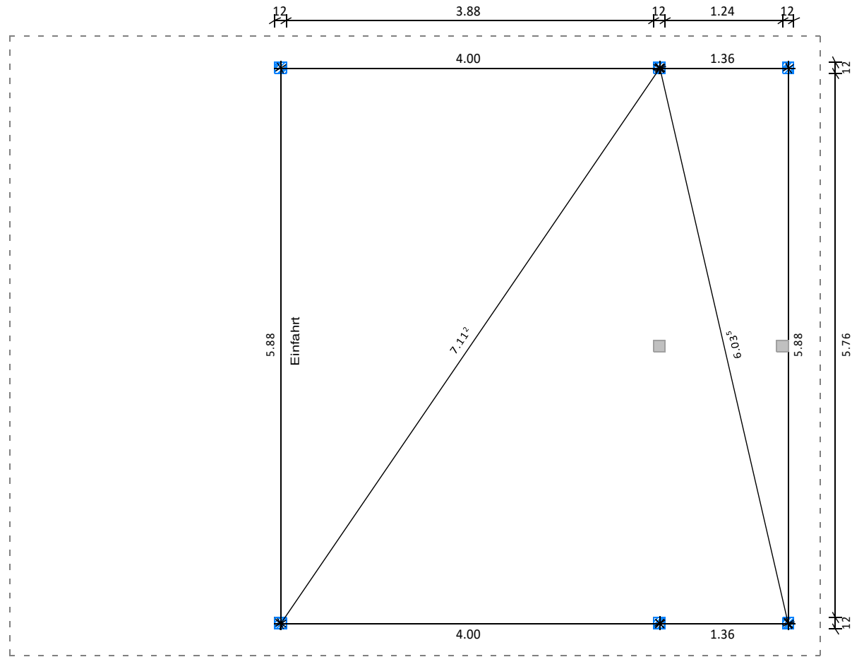
Horizontalschnitt: Pfostenmitte
