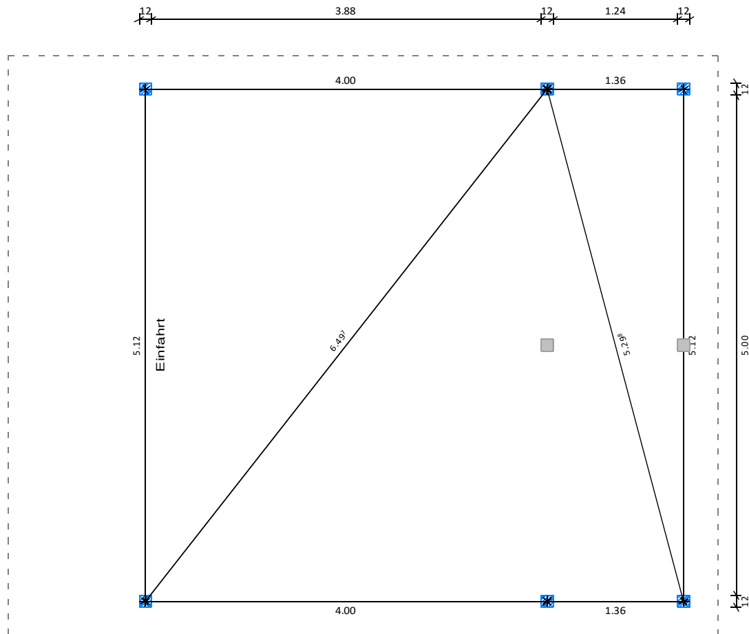
Horizontalschnitt: Pfostenmitte
