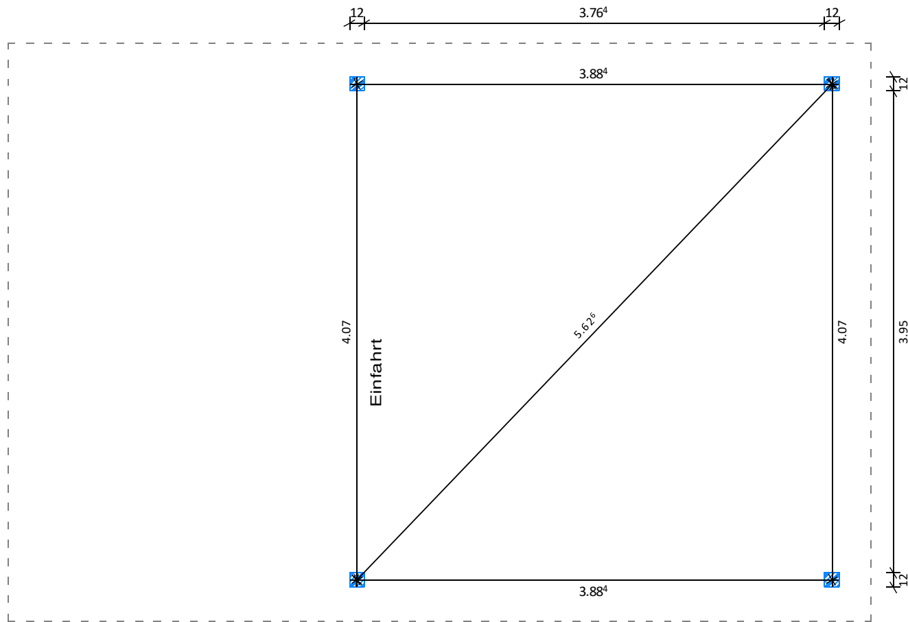
Horizontalschnitt: Pfostenmitte
