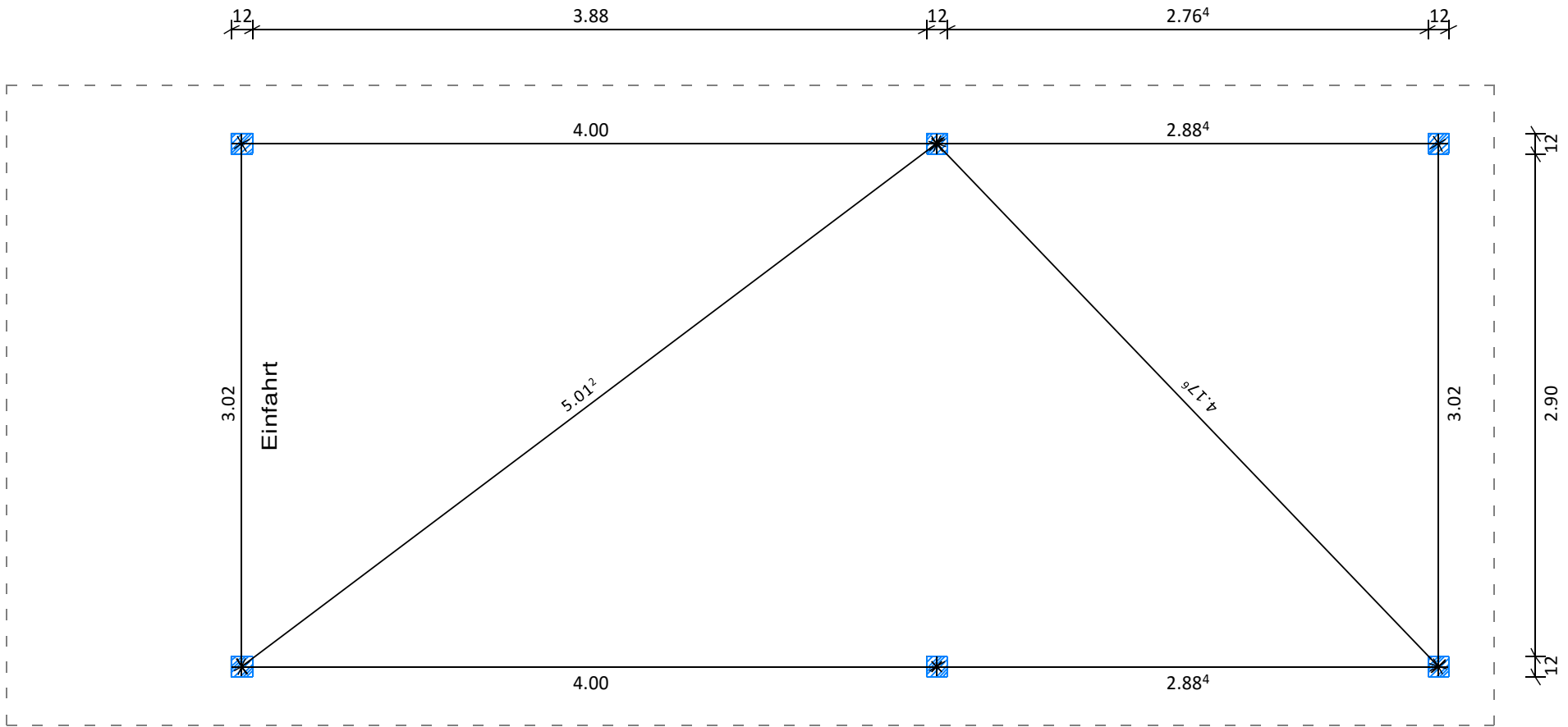
Horizontalschnitt: Pfostenmitte
